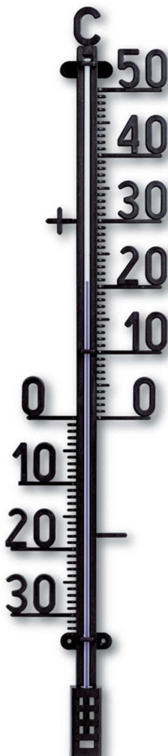
12.6005 Außenthermometer Kunststoff, schwarz, mit Befestigungsmaterial ☞ 147 x 38 x 685 mm, 167 g, 10 SB
